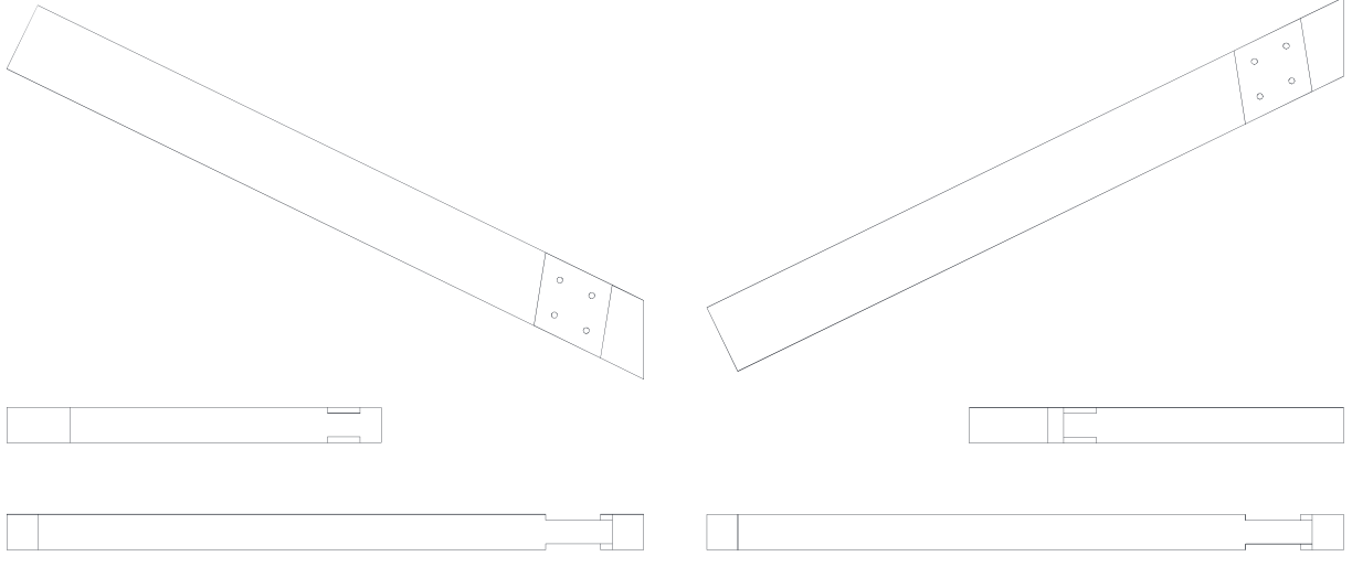
MONOLOG LOG-Steher 1:20
